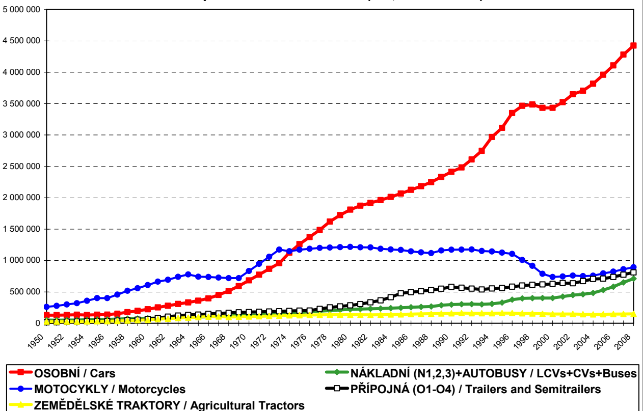
Vývoj celkového počtu registrovaných vozidel (ČR, 1950 - 2008) Development of Vehicle Parc (CR, 1950 - 2008)
